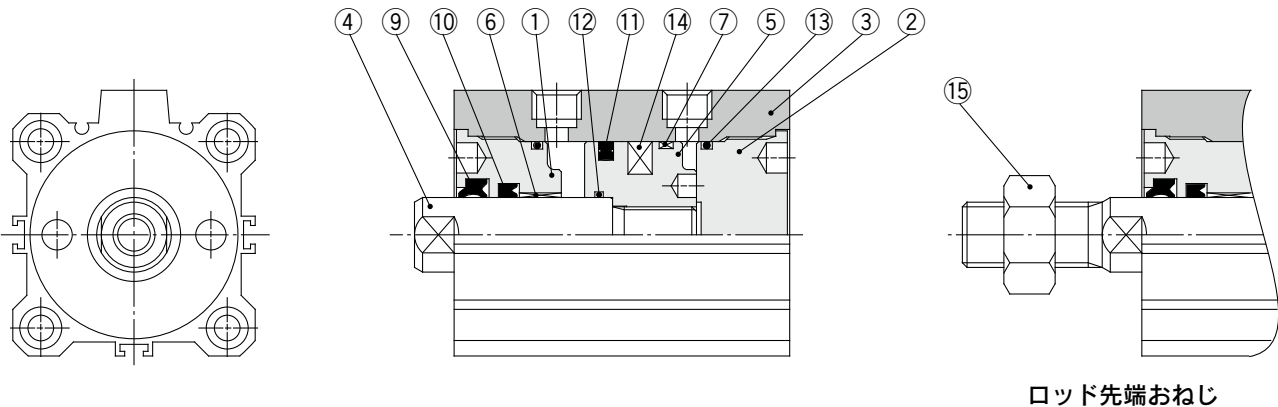
ロッド先端おねじ
