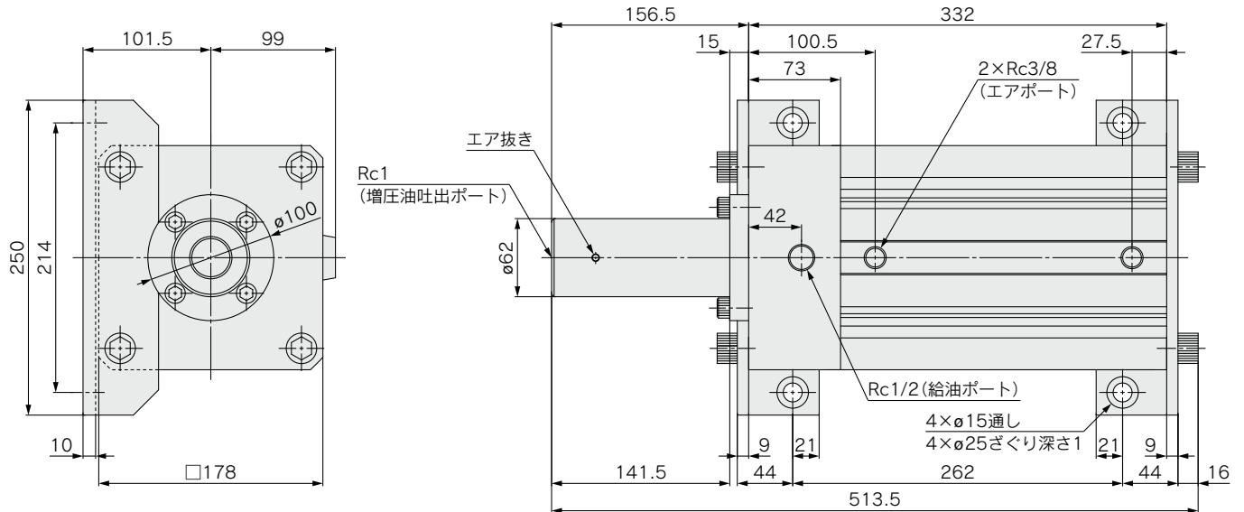
CQ2LH100-60Z-DCN5997N (増圧比1:13)/壁取付けタイプ
