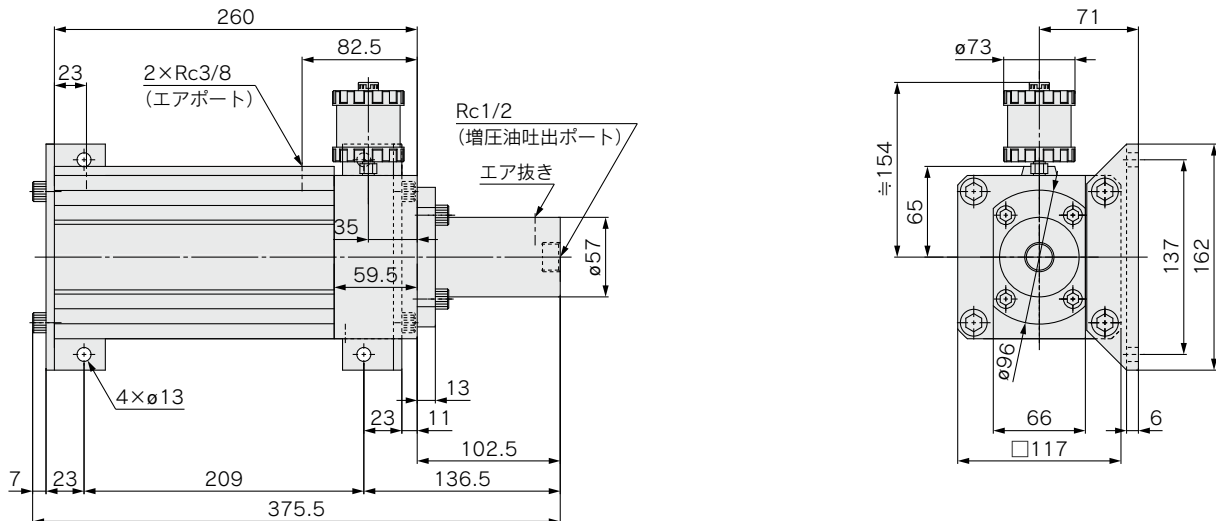
CQ2LH140-17Z-DCQ223CQ (増圧比1:15)/壁取付けタイプ
