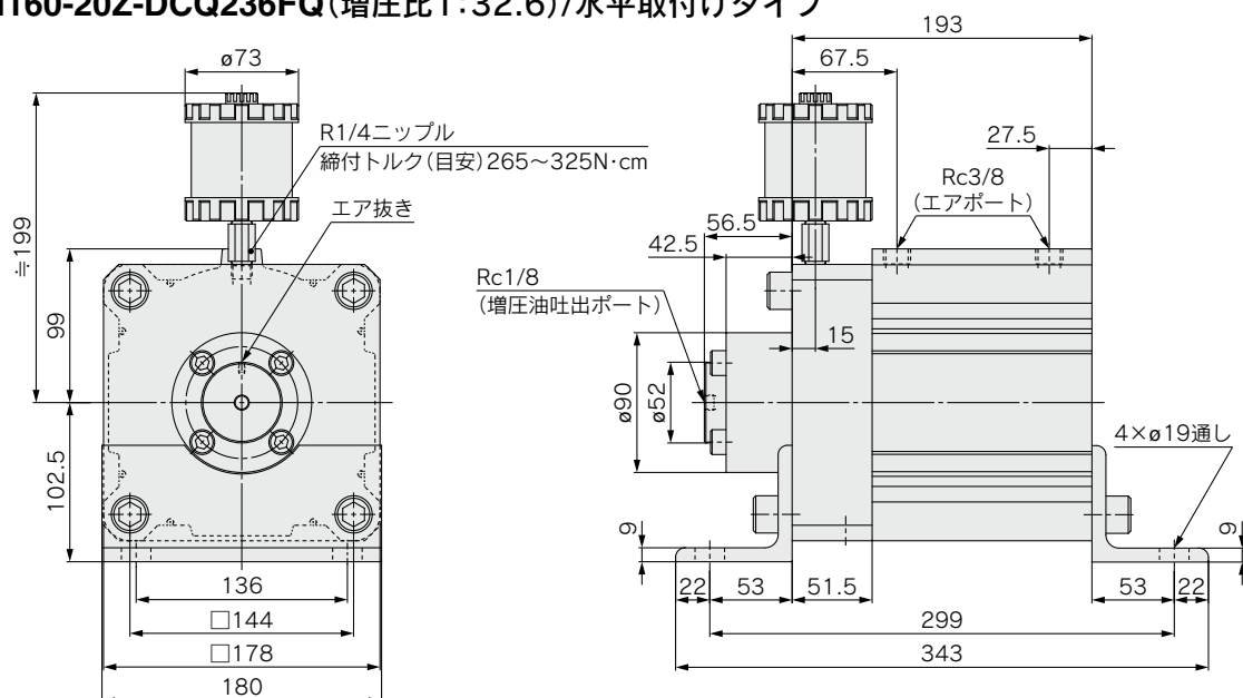
CQ2LH160-20Z-DCQ236FQ (増圧比1:32.6)/水平取付けタイプ
