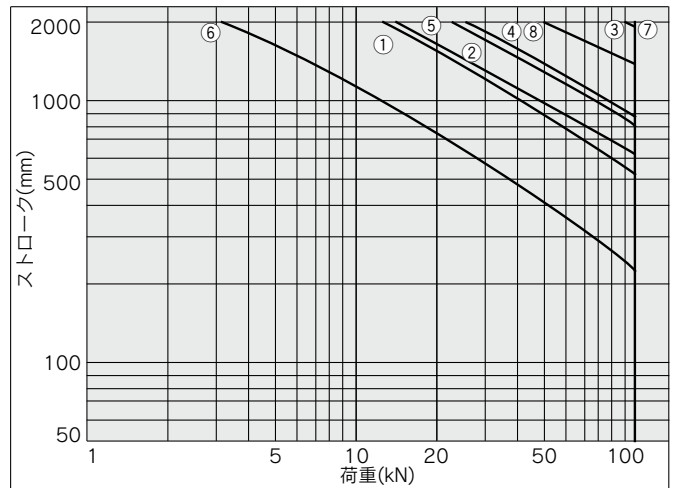
チューブ内径 \phi 100
