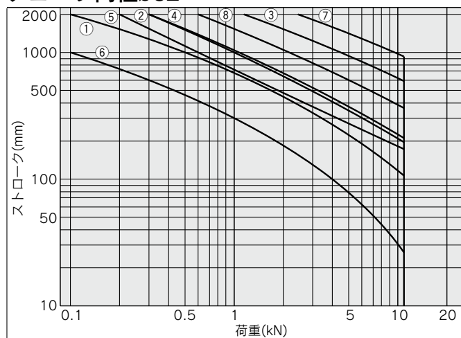
チューブ内径 \phi 32
