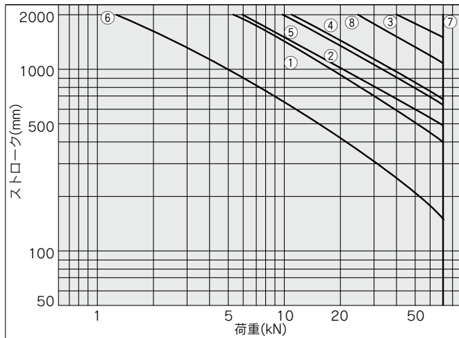
チューブ内径 \phi 80
