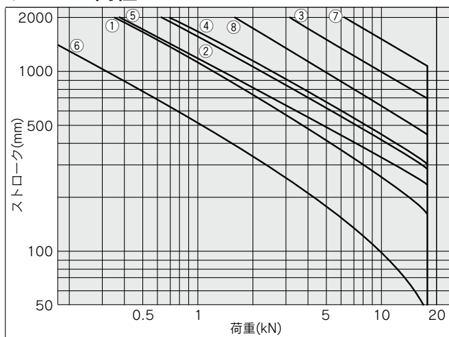
チューブ内径 \phi 40
