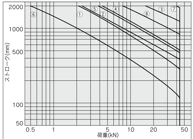
チューブ内径 \phi 63
