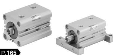
JIS規格準拠薄形油圧シリンダ CHKD Series
