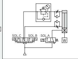
ロック付シリンダ(当社CN□シリーズ)
