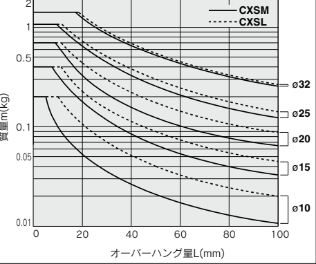
グラフ 12 V \sim 400\text{mm/s} \sim 30\text{st}
