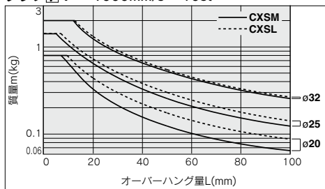
グラフ⑨ V \sim 1000\text{mm/s} \sim 30\text{st}
