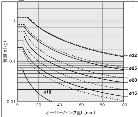
グラフ14 V=400mm/s超 ~75st
