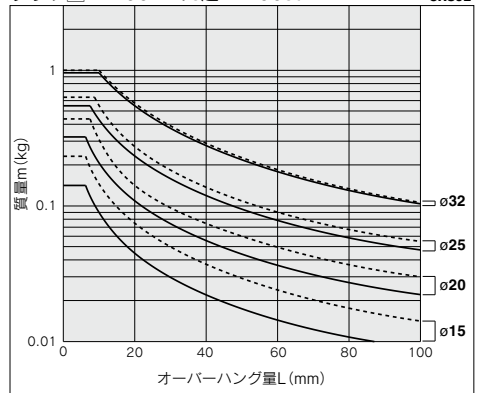
グラフ15 V=400mm/s超 ~100st
