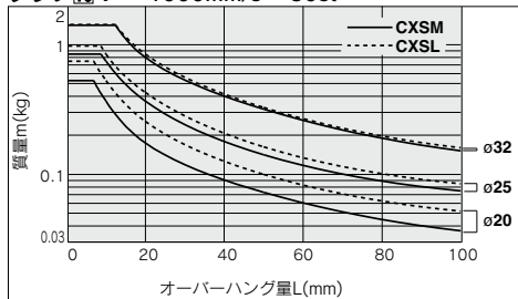
グラフ⑫ V \sim 1000\text{mm/s} \sim 100\text{st}
