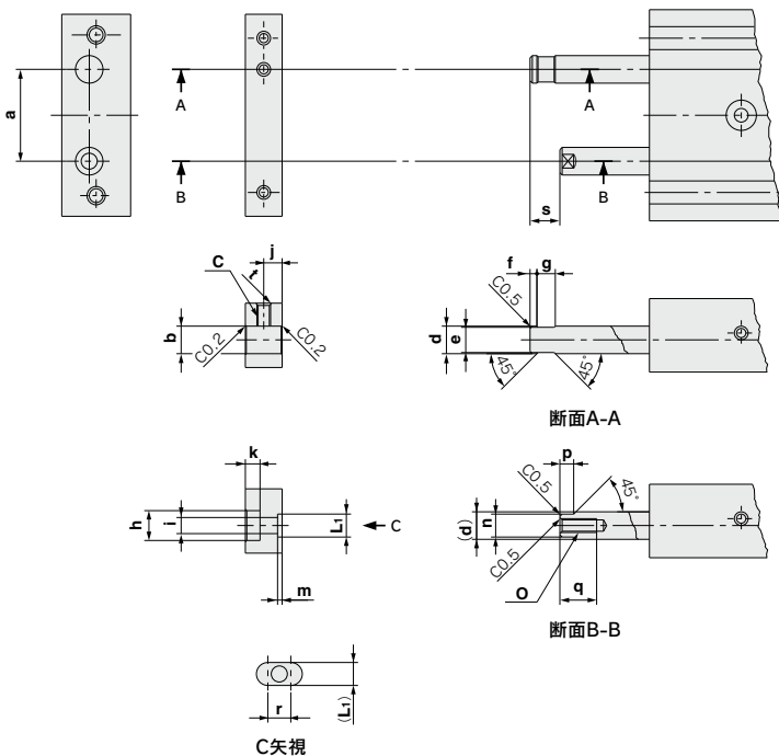
C矢視
