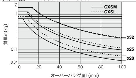
グラフ⑪ V \sim 1000\text{mm/s} \sim 75\text{st}
