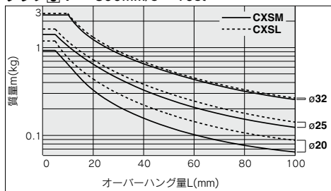
グラフ⑧ V \sim 800\text{mm/s} \sim 30\text{st}
