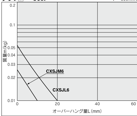
グラフ10 V=400mm/s ~30st
