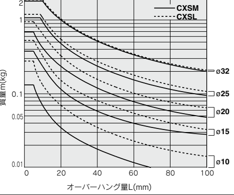
グラフ 12 V \sim 400\text{mm/s} \sim 30\text{st}
