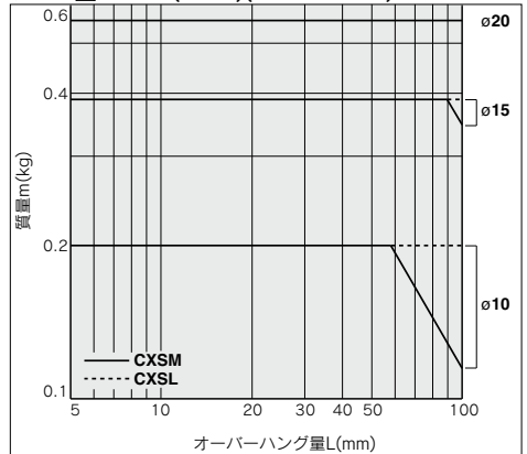
グラフ⑥ V=700(mm/s) (ø10はV=800)
